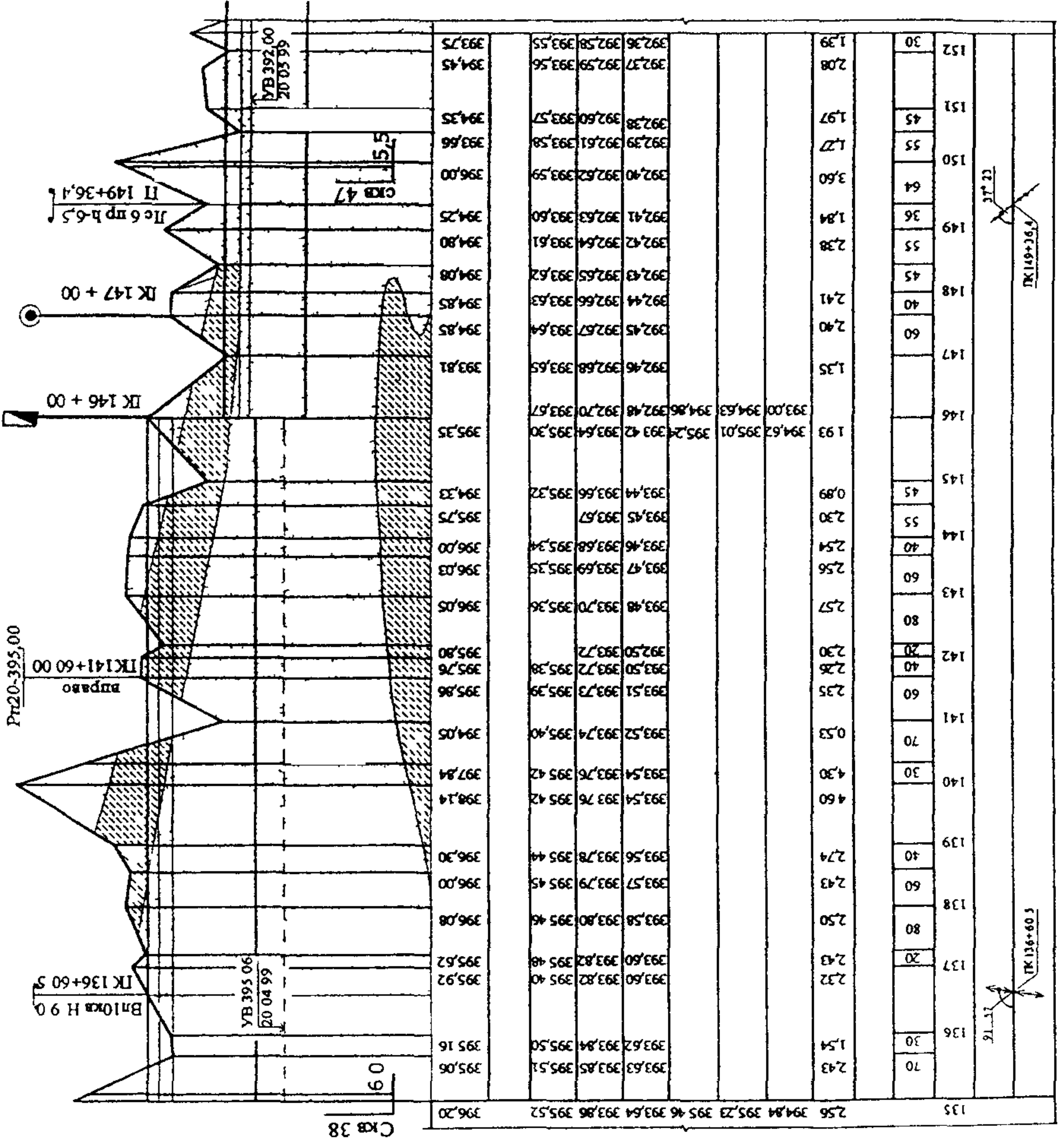
Пример оформления продольного профиля канала
